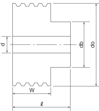
(Pulley Profile) Type B
